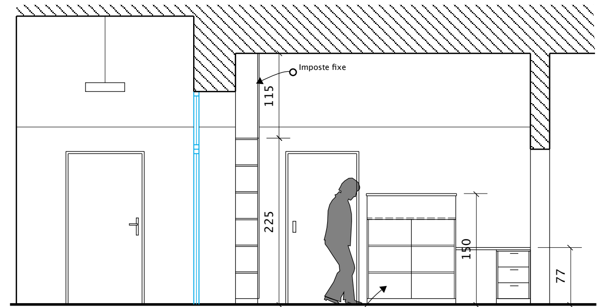
COUPE BB'
